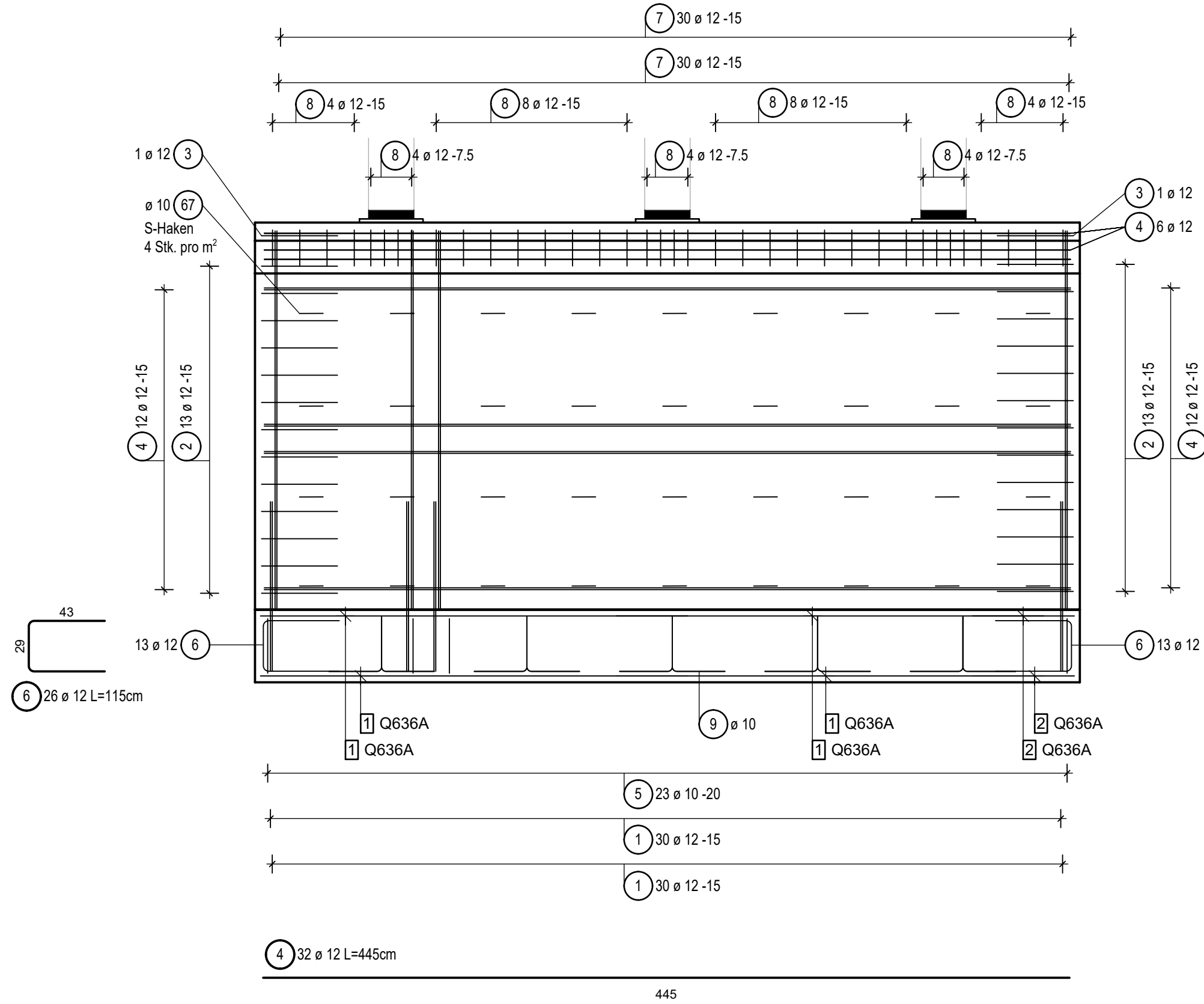
Schnitt A - A
